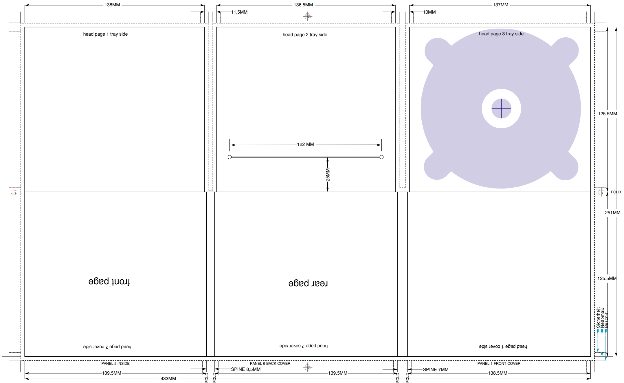
CD 6 PANEL 1 TRAY DIGIPAK mit Schlitzstanzung DBX213XX
